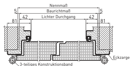
Horizontalschnitt T30-2/EI 2 30-2 / EI 2 60-2 / T90-2/EI 2 90-2
