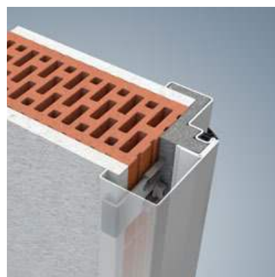
Mauerwerk verputzt
