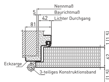
Horizontalschnitt E-S-1
