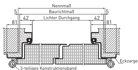
Horizontalschnitt E-S-2
