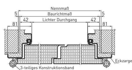
NovoPorta Premio T30-2 (EI 2 30-2)
